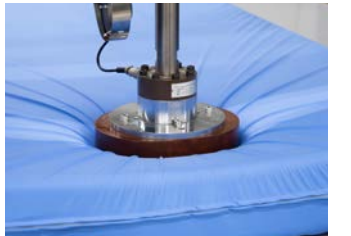
耐久試験機によるマットレスの加圧試験
